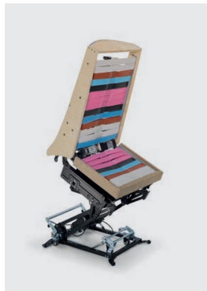
MOVIMENTO ALZAPERSONA
